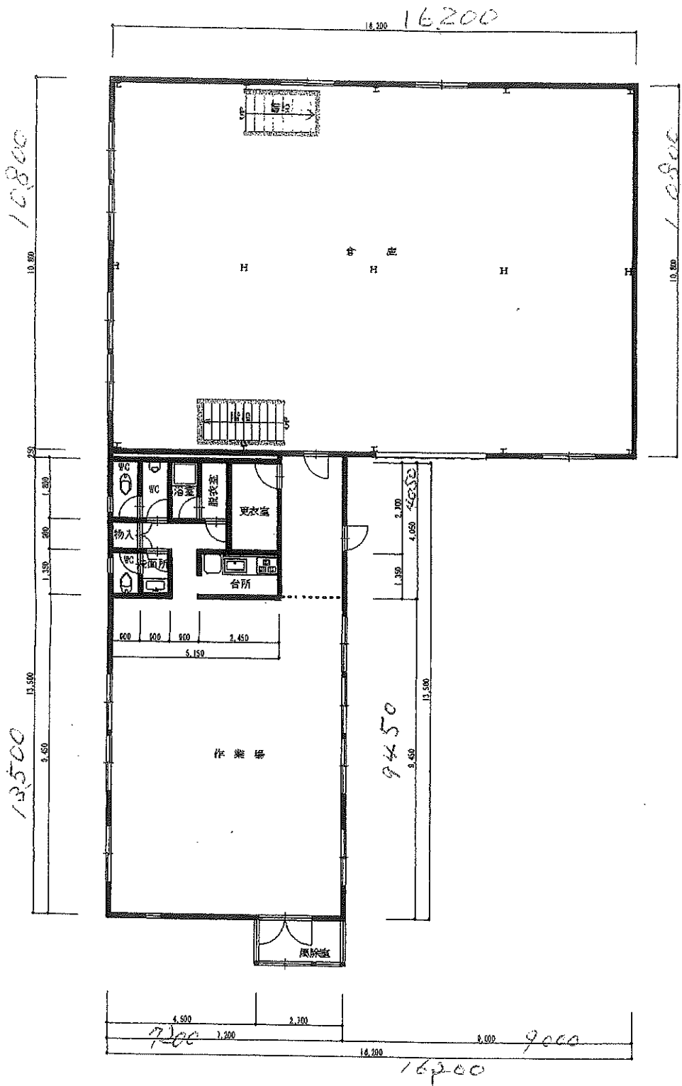
1 F 平面図
