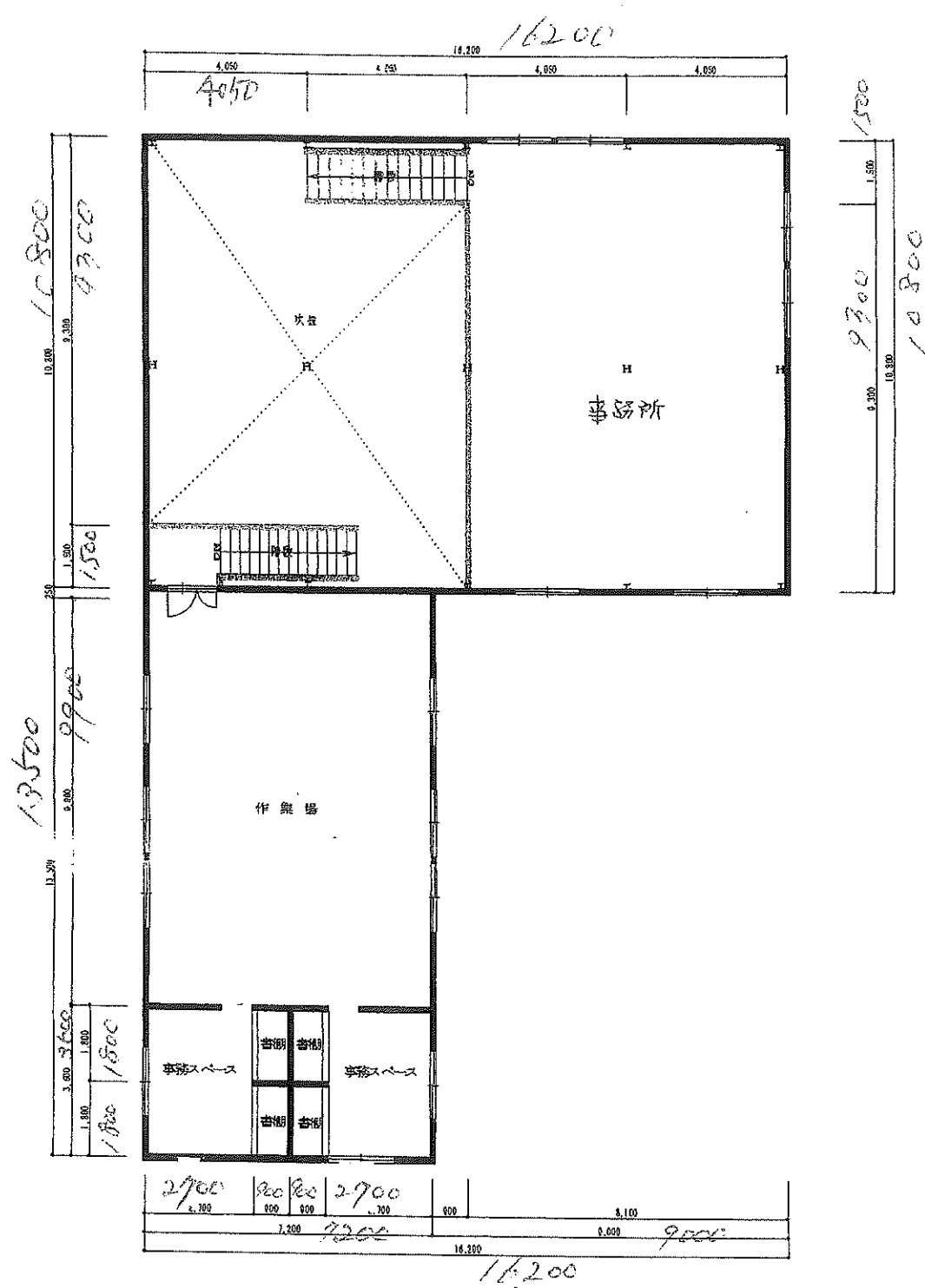
2 F 平面図
